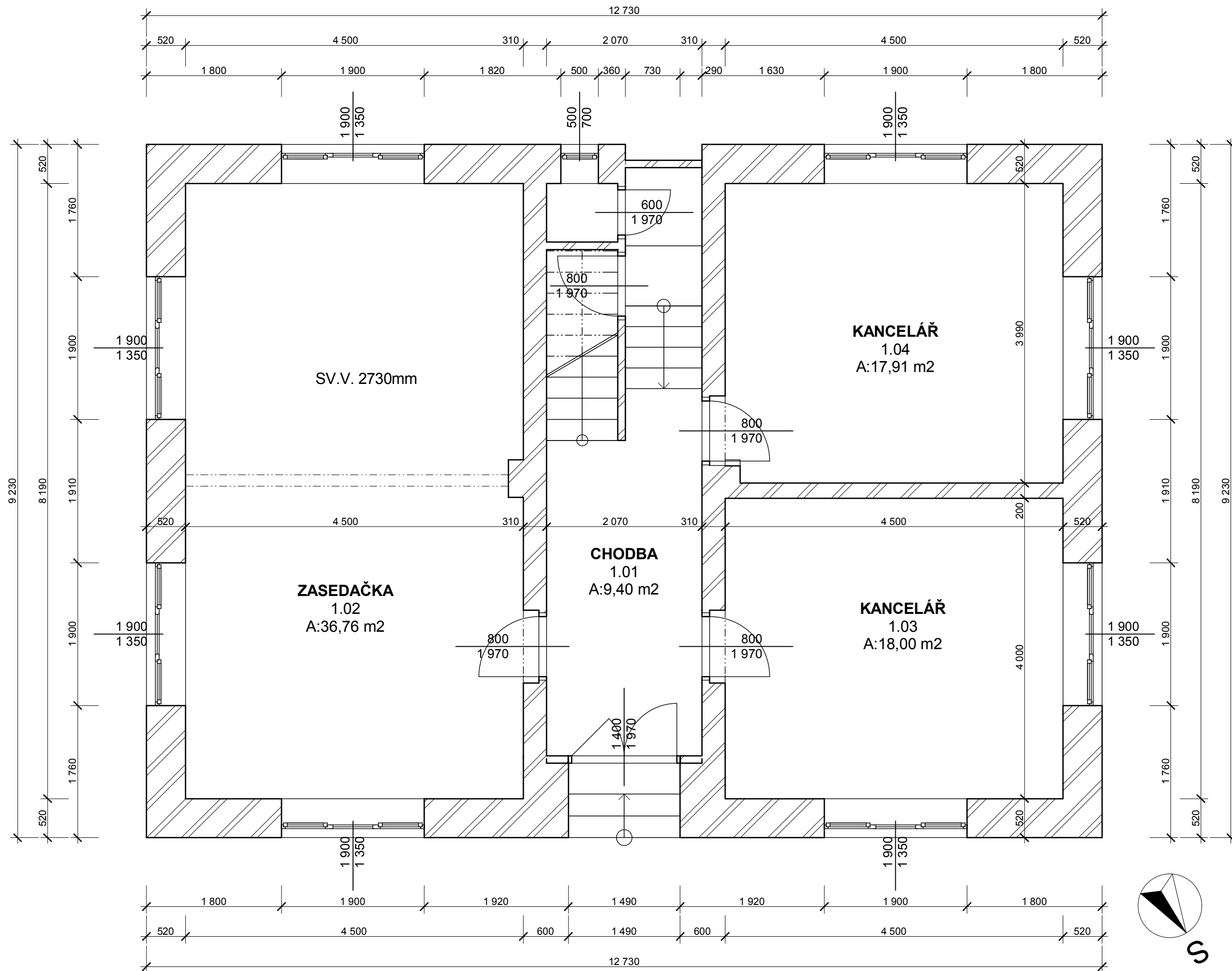
PŮDORYS- STÁVAJÍCÍ STAV 1:50
